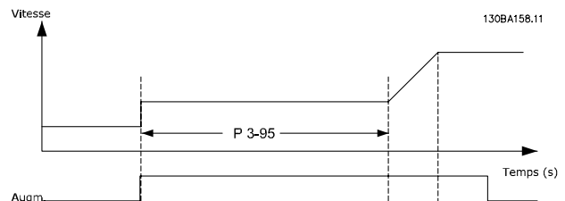
Illustration 3.29 Augmenter la référence réelle
