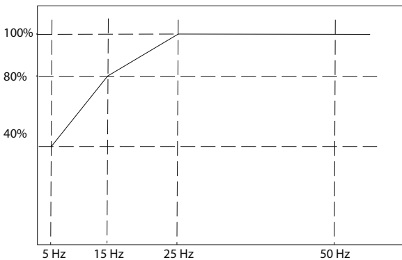
Illustration 3.18 Exemple de courbe de limite thermique ETR ATEX
