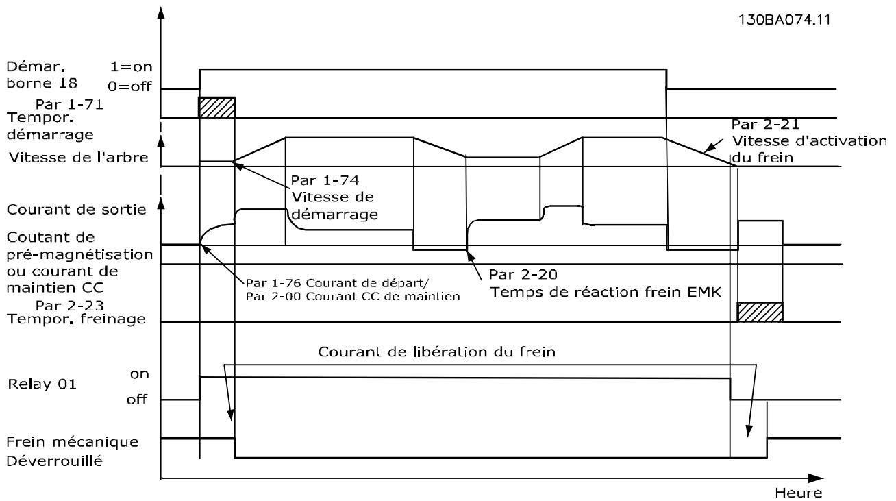
Illustration 3.19 Freinage mécanique
