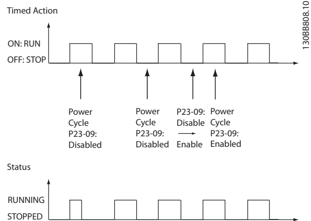
Illustration 3.70 Schéma de test de réactivation
