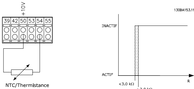
Illustration 3.14 Connexion de la thermistance PTC - entrée analogique
