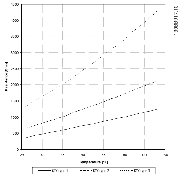
Illustration 3.15 Sélection du type KTY
