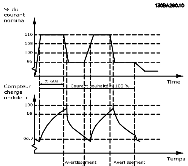
Illustration 3.64 Courant de sortie en condition de surcharge
