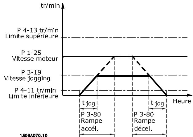
130BA070.10 Illustration 3.27 Temps de la rampe de jogging
