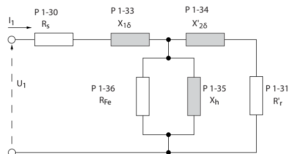
Illustration 3.6 Diagramme d'équivalence moteur pour un moteur asynchrone
