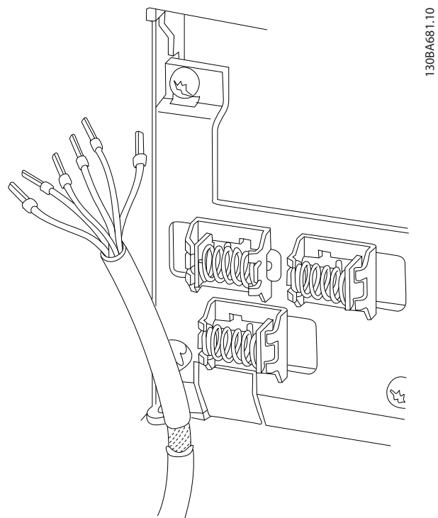
Illustration 1.5 Mise à la terre des câbles de commande blindés/armés
